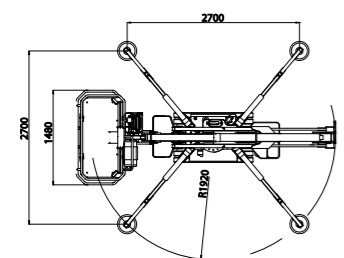
Top elevation
