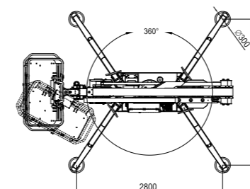
Top elevation
