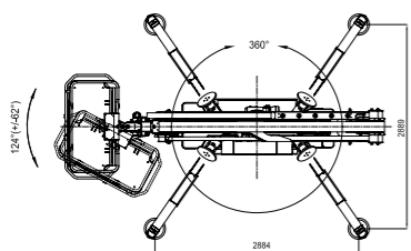
Top elevation
