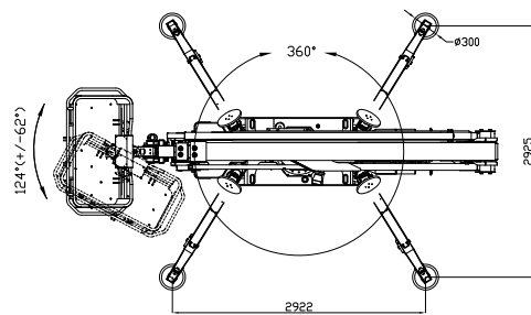
Top elevation
