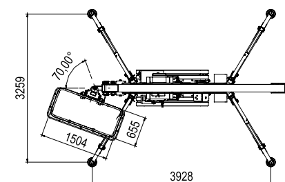
Top elevation
