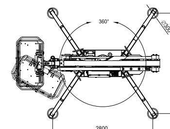
Top elevation
