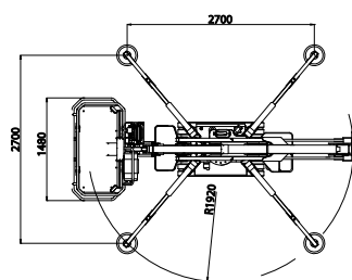
Top elevation
