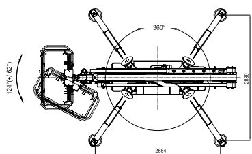
Top elevation
